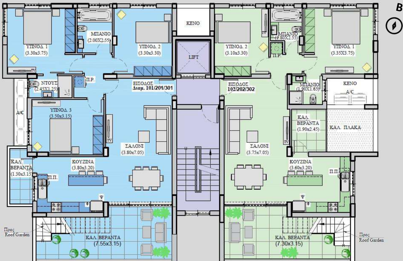
ΚΑΤΟΨΗ 4ου ΟΡΟΦΟΥ
